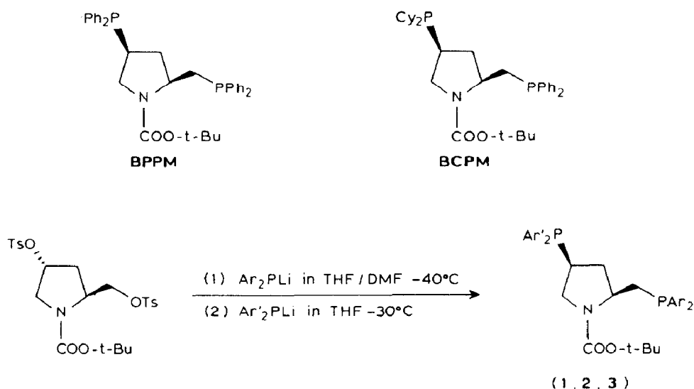
Scheme 1. 1: Ar = Ar' = p -Me 2 NC 6 H 4 , [ \alpha ] D 20 -56.6° (c 0.7, benzene); 2: Ar = Ph, Ar' = p -Me 2 NC 6 H 4 , [ \alpha ] D 20 -40.7° (c 0.7, benzene); 3: Ar = p -Me 2 NC 6 H 4 , Ar' = Ph, [ \alpha ] D 20 -45.0° (c 0.8, benzene).
