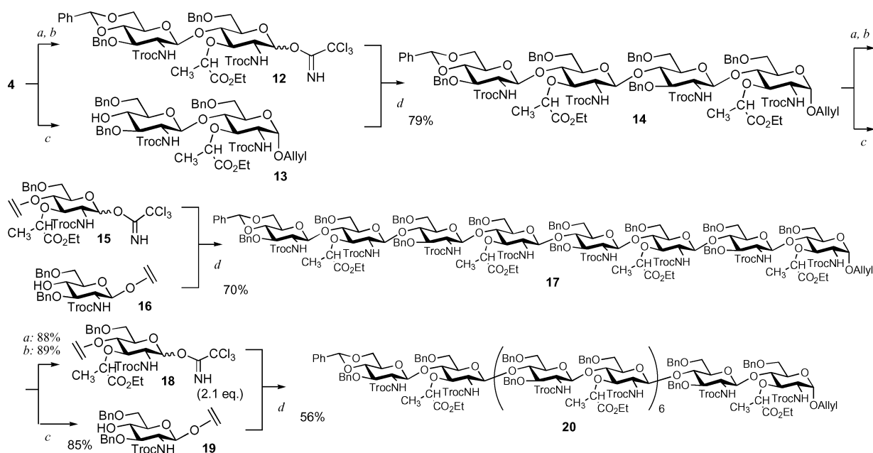
Scheme 3 Synthesis of hexadecasaccharide: (a) Ir complex, \text{H}_2 , THF, then \text{I}_2 , \text{H}_2\text{O} ; (b) \text{CCl}_3\text{CN} , \text{Cs}_2\text{CO}_3 , \text{CH}_2\text{Cl}_2 ; (c) \text{Me}_3\text{N}\cdot\text{BH}_3 , \text{BF}_3\cdot\text{Et}_2\text{O} , \text{CH}_3\text{CN} ; (d) \text{TMSOTf} (0.1 eq), MS 4A, \text{CH}_2\text{Cl}_2 , -15^\circ\text{C} .
