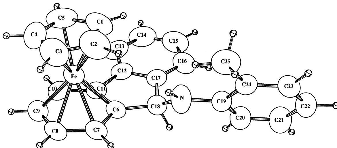
Fig. 3. ORTEP drawing of the endo isomer of 4b . Selected interatomic distances (Å): Fe–C(1) 2.023(9), Fe–C(2) 2.03(1), Fe–C(3) 2.04(1), Fe–C(4) 2.03(1), Fe–C(5) 2.04(1), Fe–C(6) 2.10(1), Fe–C(7) 2.08(1), Fe–C(8) 2.059(9), Fe–C(9) 2.071(8), Fe–C(10) 2.078(8), Fe–C(11) 2.096(9), N–C(18) 1.41(1), N–C(19) 1.38(1), N–H(26) 0.972(8).
