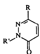
( 5 , R=Me, R'=H 6 , R=Me, R'=Me)
