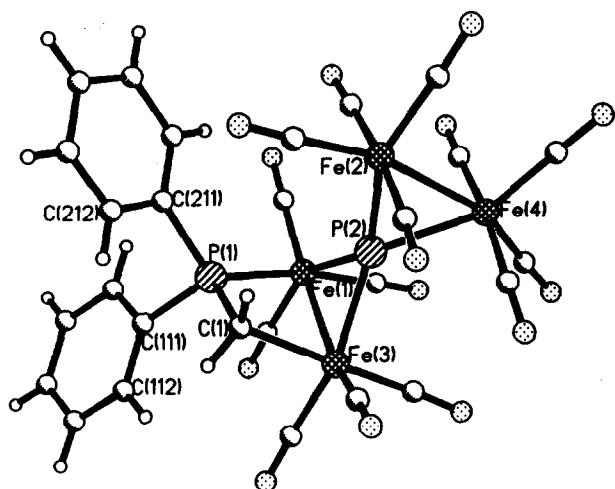
Abb. 2. Molekülstruktur von 6.
