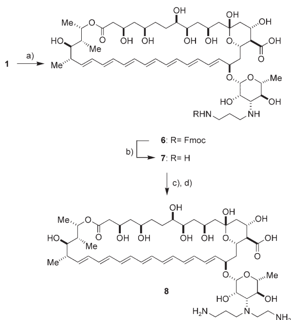
Scheme 2. a) FmocNHCH 2 CH 2 CHO, NaBH 3 CN, DMF; b) piperidine, DMSO, 7%; c) FmocNHCH 2 CHO, NaBH 3 CN, DMF; d) piperidine, DMSO, 26%.
