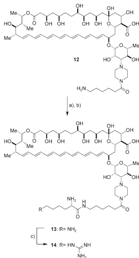
Scheme 3. a) FmocNH(CH 2 ) 4 CH(NHFmoc)CO 2 Suc, DIPEA, DMF; b) piperidine, DMSO, 28%; c) 9 , DIPEA, 20%.
