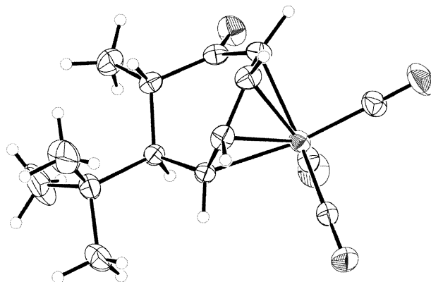
Fig. 4. ORTEP-II molecular diagram of 9f .
