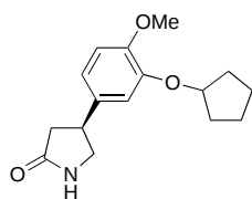
1 (+)-Rolipram
