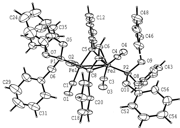
Fig. 4. ORTEX diagram of the molecular structure of 5 . Selected bond lengths (Å) and angles ( ^\circ ): \text{Fe1}-\text{Fe2} , 2.552(2); \text{Fe1}-\text{P1} , 2.105(4); \text{Fe1}-\text{C1} , 1.787(8); \text{Fe1}-\text{C2} , 1.773(8); \text{Fe1}-\text{C3} , 2.666(14); \text{Fe1}-\text{C5} , 1.988(7); \text{Fe1}-\text{C8} , 1.976(7); \text{Fe2}-\text{P2} , 2.148(3); \text{Fe2}-\text{C3} , 1.763(9); \text{Fe2}-\text{C4} , 1.757(10); \text{Fe2}-\text{C5} , 2.098(9); \text{Fe2}-\text{C6} , 2.099(9); \text{Fe2}-\text{C7} , 2.134(9); \text{Fe2}-\text{C8} , 2.159(9); \text{C5}-\text{C6} , 1.416(11); \text{C6}-\text{C7} , 1.397(10); \text{C7}-\text{C8} , 1.411(10); \text{Fe1}-\text{C5}-\text{C6} , 112.9(5); \text{C5}-\text{C6}-\text{C7} , 115.5(6); \text{C6}-\text{C7}-\text{C8} , 114.5(6); \text{C7}-\text{C8}-\text{Fe1} , 114.1(5); \text{C8}-\text{Fe1}-\text{C5} , 81.7(3); \text{P1}-\text{Fe1}-\text{Fe2} , 133.91(8); \text{C1}-\text{Fe1}-\text{C2} , 85.3(4); \text{Fe1}-\text{Fe2}-\text{P2} , 147.59(8); \text{C3}-\text{Fe2}-\text{C4} , 92.1(5).
