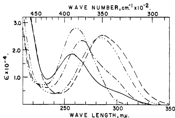
Fig. 2.—Absorption spectra of benzidines in 95% ethanol: (.....) benzidine; (---), 3,3'-dichlorobenzidine; (—) 2,2'-dichlorobenzidine; (----) 2,2'-difluorobenzidine; (-·-·-) 2,2',6,6'-tetrafluorobenzidine.
