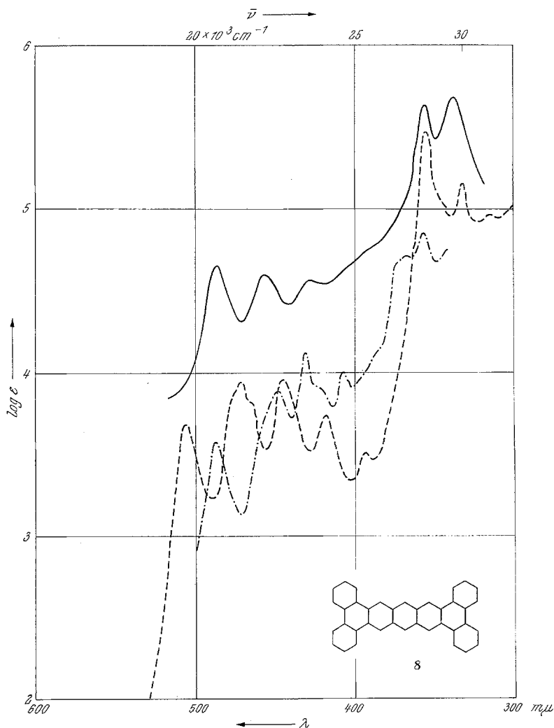
Abb. 2. Absorptionsspektrum (Maxima in m\mu ; \log \epsilon in Klammer) von: — Tetranaphthopentacen 5 in 1-Methylnaphthalin: 487 (4,64), 457 (4,60), 430 (4,56), 357 (5,62), 339 (5,67). — — — (?-Okta)-hydro-tetranaphthopentacen in 1-Methylnaphthalin: 487 (3,59), 450 (3,88), 431,5 (4,12), 407 (4,00), 367 (4,73), 357 (4,86). ····· Tetrabenzpentacen 8 in 1-Methylnaphthalin nach E. Clar, W. Kelly und W. G. Niven, J. chem. Soc. [London] 1956, 1833; ab 340 m\mu in Benzol nach Clar 7e .
