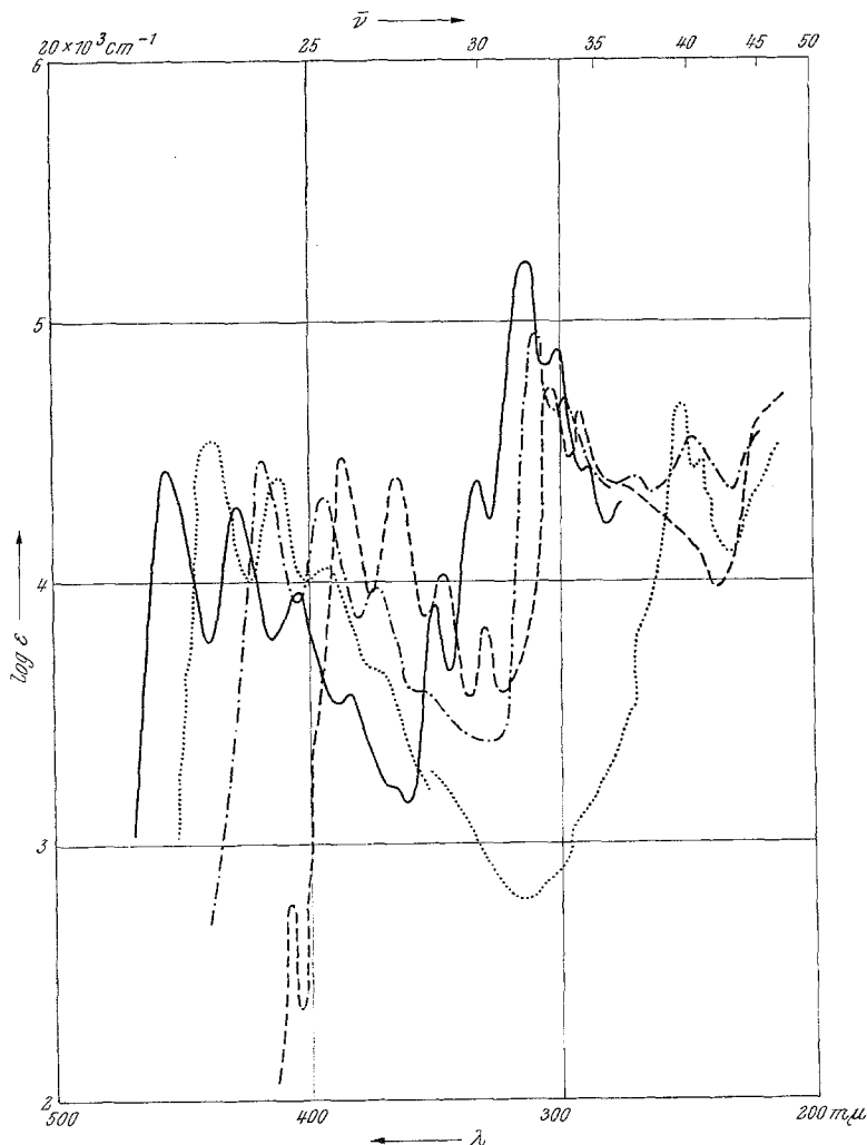
Abb. 1. Absorptionsspektrum (Maxima in m\mu ; \log \epsilon in Klammer) von: — Anthraperylen 4 in Benzol: 457 (4,43), 429 (4,29), 404 (3,96), 384 (3,58), 352 (3,91), 334 (4,38), 314 (5,25), 302 (4,89), 290 (4,42). - - - Naphthoperylen 3 in Benzol nach Clar , Ironsides und Zander 6 . ····· Benzperylene 2 in Benzol, ab 280 m\mu in Alkohol nach Clar 1 . ..... Perylen 1 in Benzol nach E. Clar , Chem. Ber. 81 , 55 (1948), ab 350 m\mu in Alkohol nach Clar 1 .
