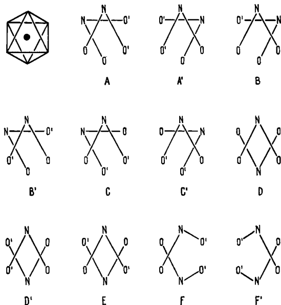
Fig. 1. Koordinations-Okttaeder um \text{Cr}^{3+} und die 11 stereomeren Anordnungen zweier dreizähliger o,o' -Dihydroxy- trans -azo-Liganden
