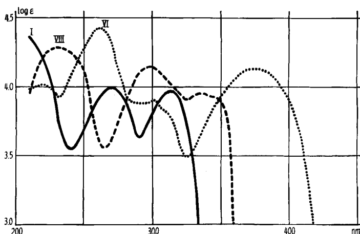
Fig. 1. UV.-Spektren von Schizozysin (I, —), Oxydationsprodukt VI aus Dihydroschizozysin (.....) und Schizozysinisomethin (VIII, - - -)
