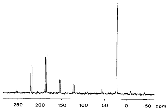
Fig. 5. ^{13}\text{C} CP-MAS NMR spectrum of \text{Y}(\text{CH}_3\text{CO}_2)_3 \cdot 4\text{H}_2\text{O} .
