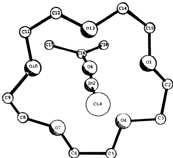
Fig. 3. The structure of the cation [\text{ZnCl} \cdot 15\text{-crown-5} \cdot \text{CH}_3\text{COCH}_3]^+ in the complex salt [\text{ZnCl} \cdot 15\text{-crown-5} \cdot \text{CH}_3\text{COCH}_3]_2^+[\text{Zn}_2\text{Cl}_6]^{2-} (IV).
