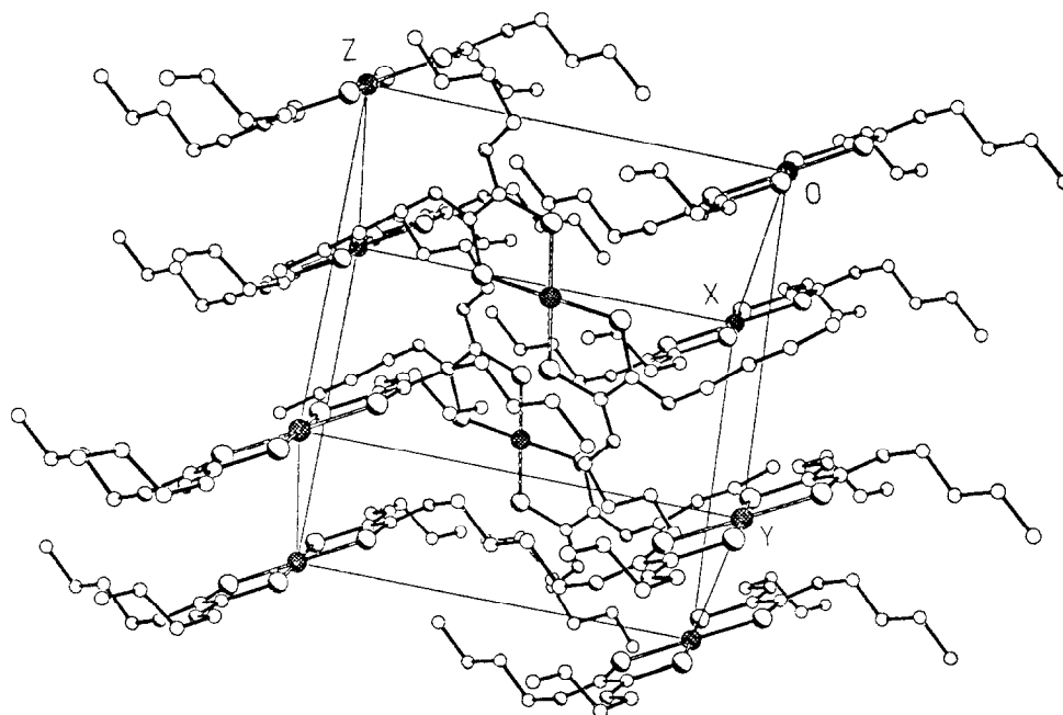
Fig. 3. Molecular packing of [Pt(H- n bu 2 -DTO) 2 ].
