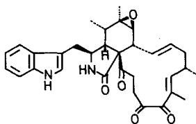
Chaetoglobosin C ( 3 )
