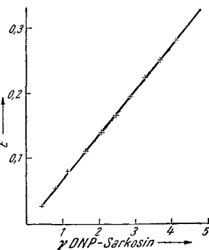
Abb. 5. Eichkurve für DNP-Sarkosin bei Wellenlänge 390 m\mu und dem Salzgehalt des Versuches.
