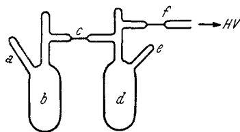
Abb. 2. Apparatur zur Hochvakuumzersetzung des Sarkosin-N-carbonsäureanhydrids.
