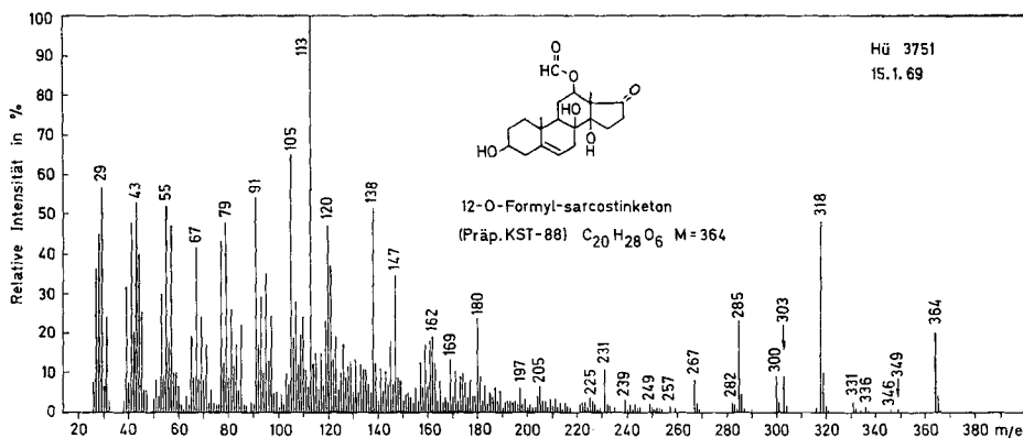
Fig. 4. Massenspektrum von 12-O-Formyl-sarcostinketon (4), Präp. KST-88, amorph Versuchsweise Zuordnung: 364 = M ; 349 = M - \text{CH}_3 ; 346 = M - \text{H}_2\text{O} ; 336 = M - \text{C}_2\text{H}_4 oder M - \text{CO} ; 331 = M - \text{CH}_3 - \text{H}_2\text{O} ; 318 = M - 46(\text{HCOOH}) ( m^* ber.: 277,8; gef.: 278); 303 = 318 - \text{CH}_3 ; 300 = 318 - \text{H}_2\text{O} ( m^* ber.: 283,0; gef.: 283); 285 = 318 - \text{CH}_3 - \text{H}_2\text{O} ; 267 = 285 - \text{H}_2\text{O} ( m^* ber.: 250,1; gef.: 250,5). Weitere Spitzen vgl. KAPUR et al. [9].
