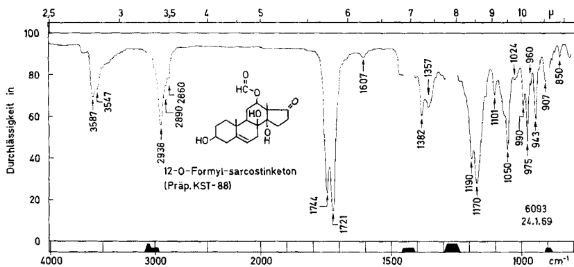
Fig. 3. IR-Absorptionsspektrum von 12-O-Formyl-sarcostinketon (4) amorph, c = 0,06 molar in \text{CH}_2\text{Cl}_2 -Lösung, d = 0,2 \text{ mm}^3 )
