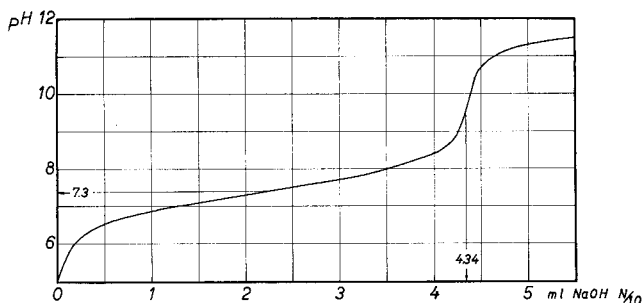
Fig. 9. Potentiometrische Titration von 1-Phenylcarbamyl-4,4-diäthyl-3-Pyrazolidinon (pH/ml)
