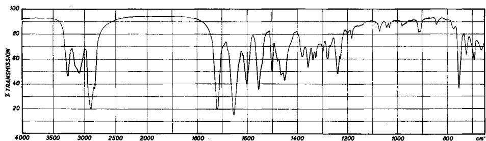
Fig. 5. IR.-Spektrum von 1-Phenylcarbamyl-4,4-diäthyl-3-pyrazolidinon in Nujol
