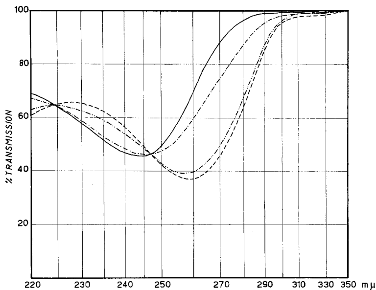
Fig. 8. UV.-Spektren bei verschiedenen pH-Werten von 1-Phenylcarbamyl-4,4-diäthyl-3-pyrazolidinon ( E/m\mu )
