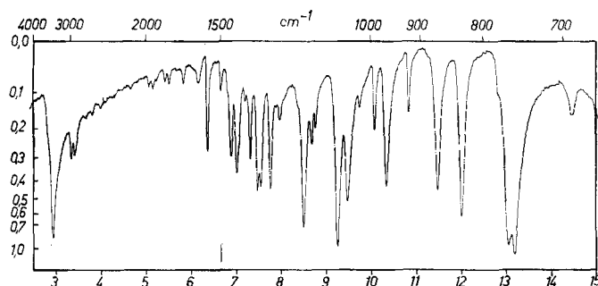
Fig. 2. 2-(2-Hydroxyäthyl)-benzotriazol
