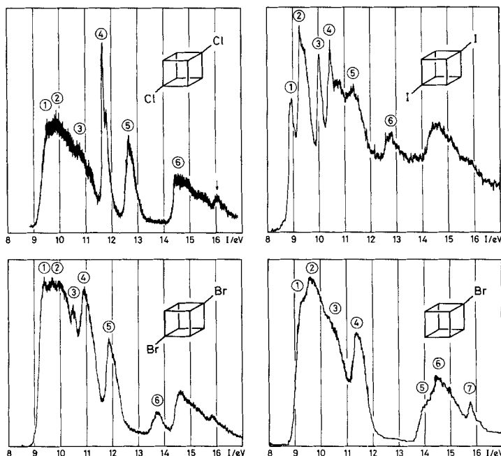
Fig. 1. \text{He}(I\alpha) PE Spectra of 2-5
