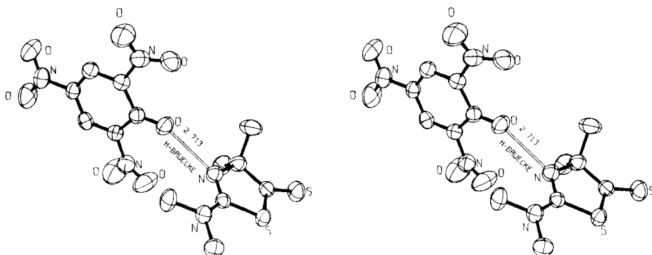
Fig. 2. Stereoprojektion von 17-Pikrat
