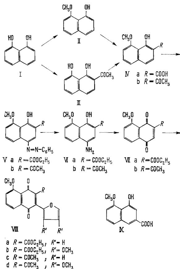
Formelschema 1
