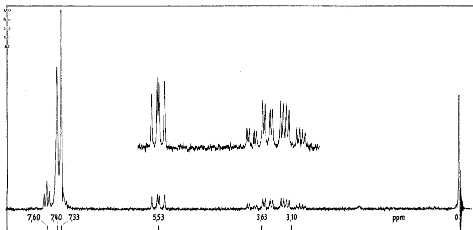
Fig. 2. NMR.-Spektrum von Verbindung XXIV in \text{CDCl}_3
