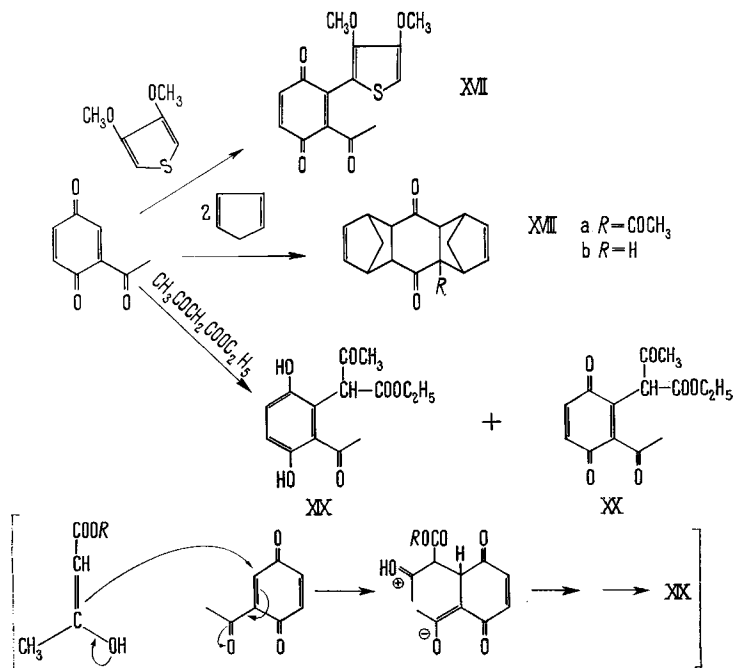
Formelschema 3
