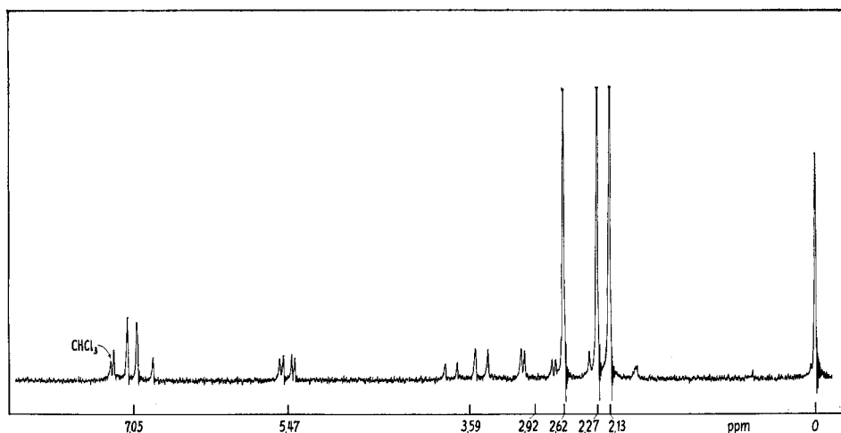
Fig. 1. NMR.-Spektrum von Verbindung XXII in \text{CDCl}_3
