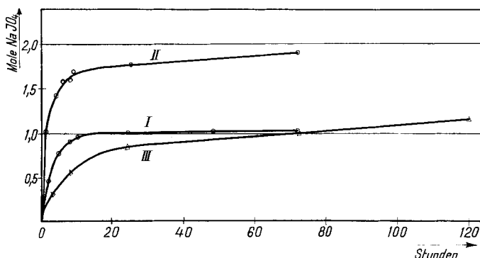
Fig. 2. Perjodatoxydationen bei 22°
