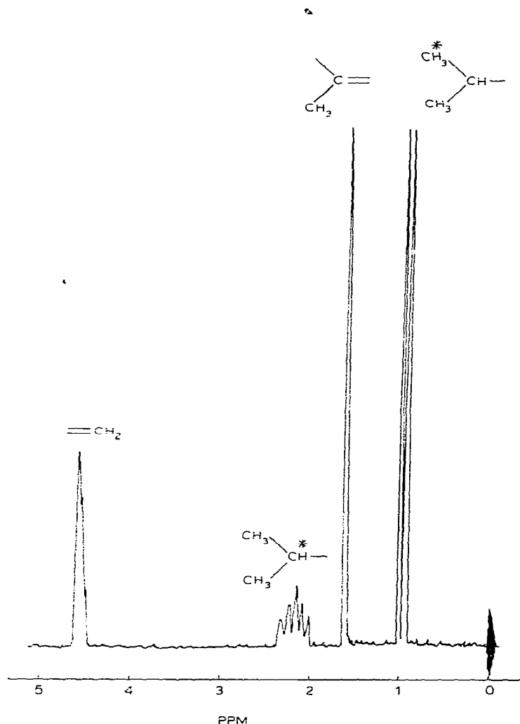
Fig. 5. 90 Mc ^1\text{H} spectrum of (\text{CH}_3)_2\text{CHC}=\text{CH}_2 .
