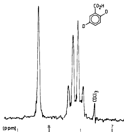
Fig. 3. ^1\text{H} -NMR. spectrum of 2,5-dideuteriobenzoic acid ( \text{CDCl}_3 )
