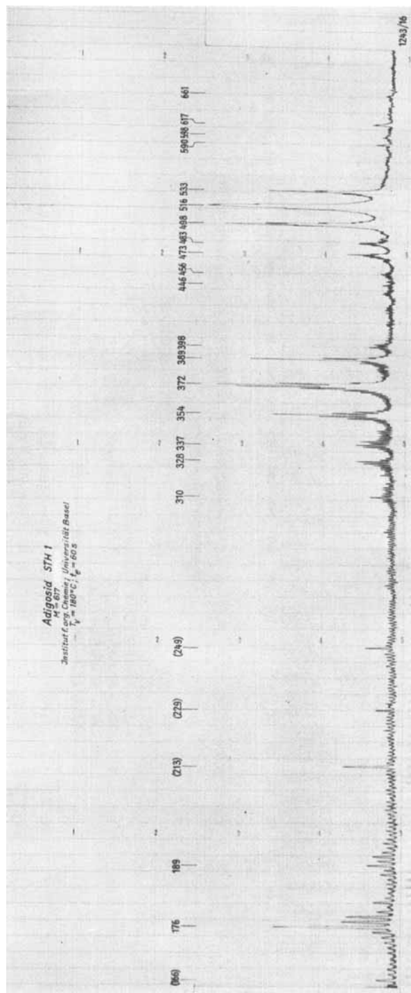
Fig. 1. Anionen-Massenspektrum von Adigosid (2) (Präp. STH 1), Smp. 141-145^\circ/158^\circ 18)
