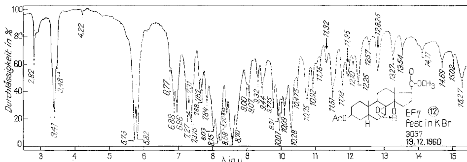
Fig. 7. IR.-Absorptionsspektrum von 3 \beta -Acetoxy-7,8 \beta -epoxy-14 \beta -hydroxy-5 \beta -ätiansäure-methylester 12 , fest, 1,8 mg in ca. 300 mg KBr 15)16) (vgl. auch Fig. 2 und 3) – Eine Esterbande (5,73 \mu ) unverbrückt, eine zweite (5,82 \mu ) assoziiert. In CH 2 Cl 2 (Nr. 3417) ist nur eine Bande bei 5,79 \mu sichtbar.
