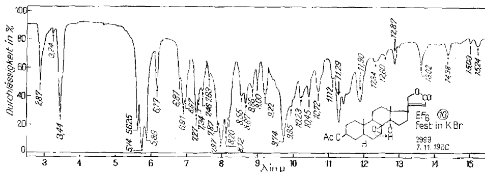
Fig. 6. IR.-Absorptionsspektrum von 3-O-Acetyl-tanghinigenin 10, fest, 1,8 mg gepresst in ca. 300 mg KBr 15) 16)
