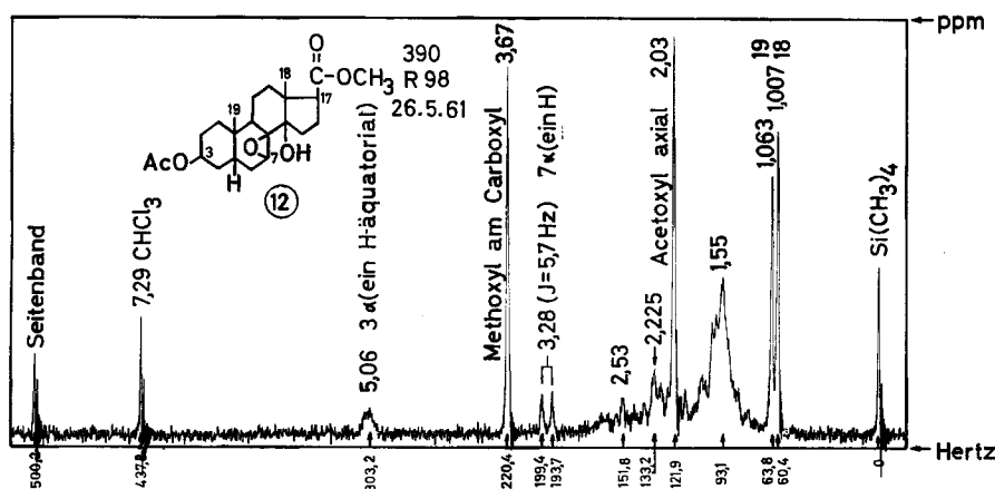
Fig. 16. Protonenresonanzspektrum von 3β-Acetoxy-7,8β-epoxy-14β-hydroxy-5β-ätiensäure-methylester 12 , 15,6 mg in 0,4 ml \text{CDCl}_3 17)
