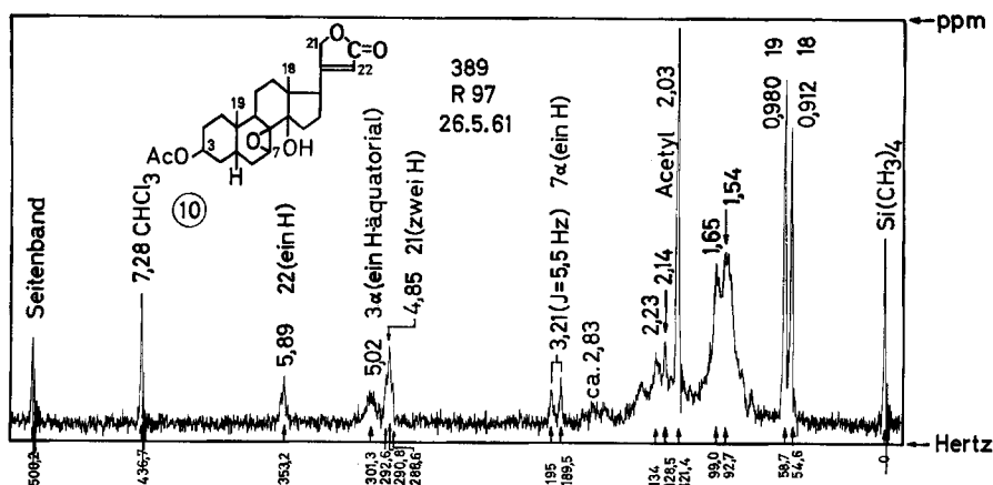
Fig. 15. Protonenresonanzspektrum von 3-O-Acetyl-tanghinigenin 10 , 16,1 mg in 0,39 ml \text{CDCl}_3 17)
