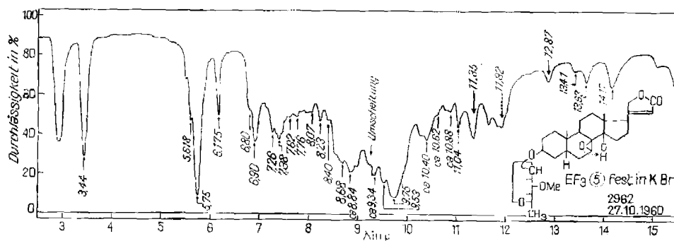
Fig. 4. IR.-Absorptionsspektrum von Desacetyltanghinin 5, 2 mg gepresst in ca. 300 mg KBr 15) 16)
