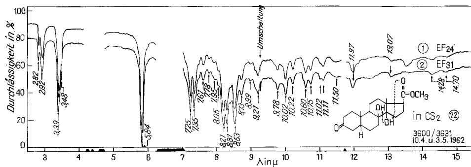
Fig. 11. IR.-Spektren von 3-Oxo-8 \beta ,14 \beta -dihydroxy-5 \beta -ätiensäure-methylester 22 , c = 0,06 \text{ M} in CS 2 , d = 0,2 \text{ mm}^{12} )
