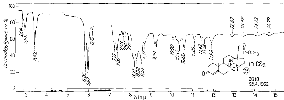
Fig. 13. IR.-Spektrum von 3-Oxo-8 \beta ,14 \beta -dihydroxy- \Delta^4 -ätiensäure-methylester 26 , gesättigte Lösung (ca. 0,06 M) in CS 2 , d = 0,2 \text{ mm}^{12)}
