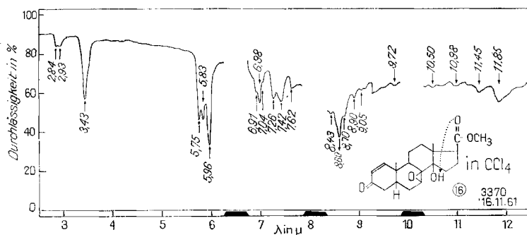
Fig. 12. IR.-Spektrum von 3-Oxo-7,8 \beta -epoxy-14 \beta -hydroxy- \Delta^1 -5 \beta -ätiensäure-methylester 16 , gesättigte Lösung in CCl 4 , d = 0,2 \text{ mm}^{12} )
