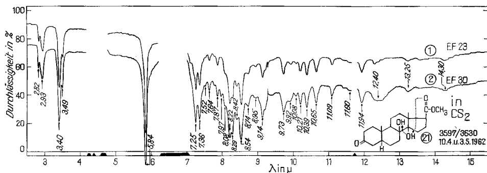
Fig. 10. IR.-Spektren von 3-Oxo-8 \beta ,14 \beta -dihydroxy-5 \alpha -ätiensäure-methylester 21 , gesättigte Lösung (ca. 0,06 M) in CS 2 , d = 0,2 \text{ mm}^{12} )
