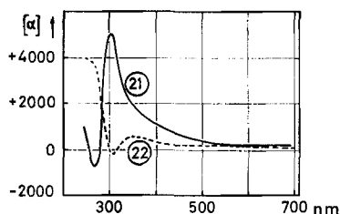
Fig. 18. Rotationsdispersion 20)
