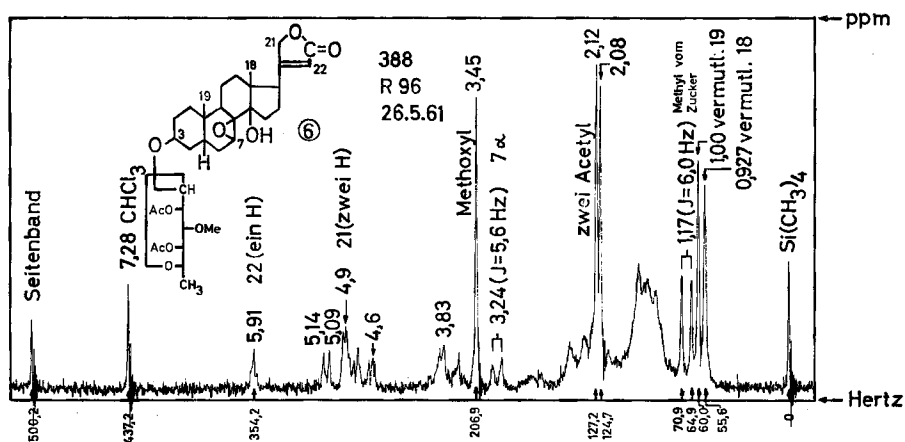
Fig. 14. Protonenresonanzspektrum von O-Acetyl-tanghinin 6 , 16,0 mg in 0,3 ml CDCl 3 17)
