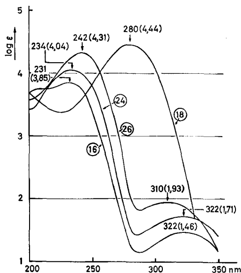
Fig. 17. UV-Absorptionsspektren in Alkohol 19)
