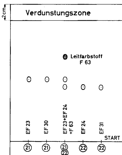
Fig. 20. Beispiel eines Dünnschichtchromatogramms nach der Durchlaufmethode [25], Fließmittel: Petroläther-Äther-(1:1), F 63 = Leitfarbstoff = 1-(o-Methoxybenzol)-azo-2-naphtol
