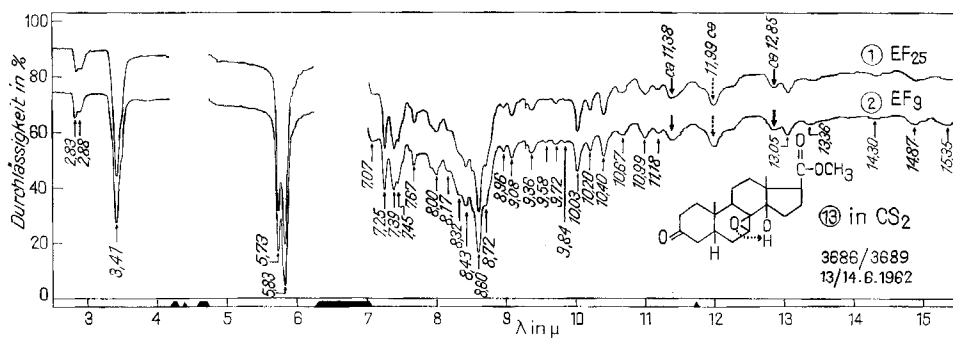
Fig. 8. IR.-Absorptionsspektren von 3-Oxo-7,8 \beta -epoxy-14 \beta -hydroxy-5 \beta -ätiansäure-methylester 13 , gesättigte Lösung ( c = \text{ca. } 0,06 \text{ M} , d = 0,2 \text{ mm} in CS 2 12)16)
