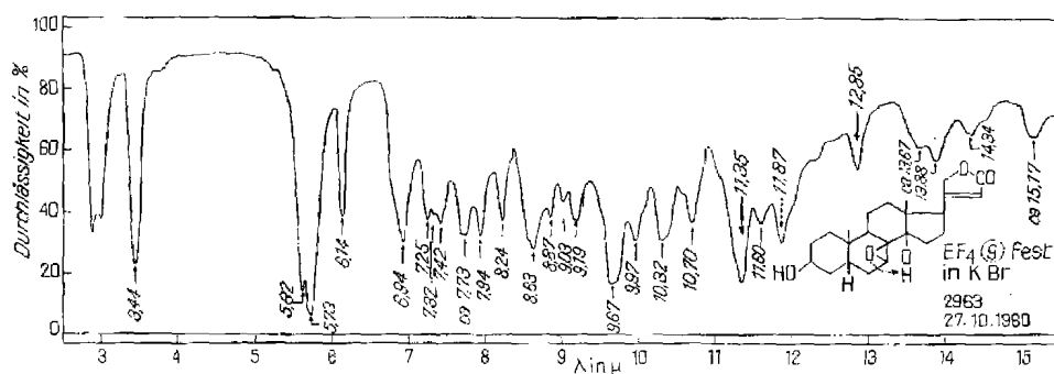
Fig. 5. IR.-Absorptionsspektrum von Tanghinigenin 9, fest, 2 mg gepresst in ca. 300 mg KBr 15) 16)
