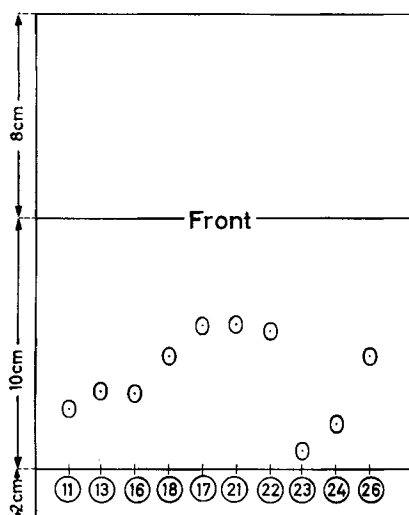
Fig. 19. Beispiel eines Dünnschichtchromatogramms [24], Fließmittel: Äther
