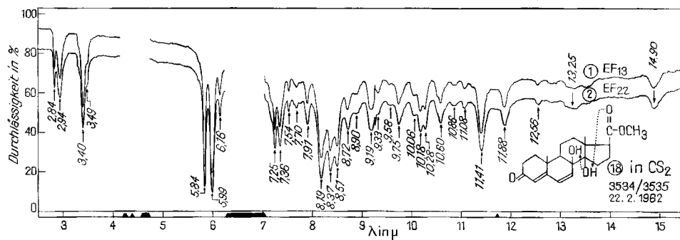
Fig. 9. IR.-Spektren von 3-Oxo-8 \beta ,14 \beta -dihydroxy-ätia-4,6-dien-säure-methylester 18 , gesättigte Lösung (ca. 0,05 M) in CS 2 , d = 0,2 \text{ mm} 12)
