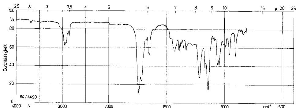
Fig. 4. IR.-Absorptionsspektrum des Ketoesters 13 in Methylenchlorid 7)
