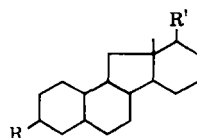
2, R, R' = O-funktionelle Gruppen
