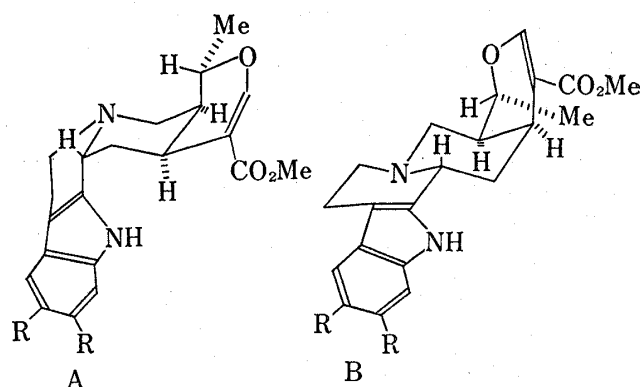
13 : R=H 20 : R=OMe
