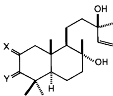
2 X = H 2 , Y = O
