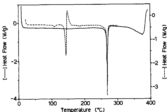
Fig. 2. DSC curves of Mo(CO) 5 (dppf) (-----) and Mo(CO) 4 (dppf) (——).
