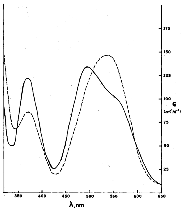
Figure 5. Visible spectra of IV (—) and VI (---).
