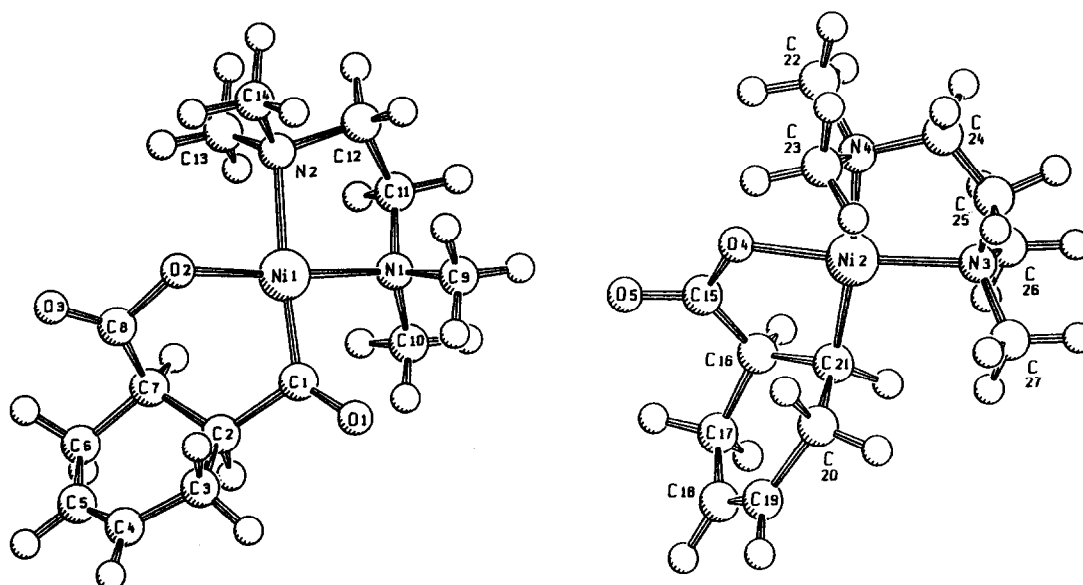
Abb. 2. Strukturen des Acyl-Nickelkomplexes 2 und des Nickelalactons 4.
