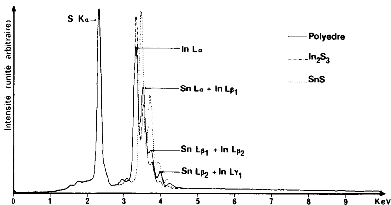
FIG. 2. Spectre de microanalyse qualitative par sonde électronique relatif aux polyèdres.
