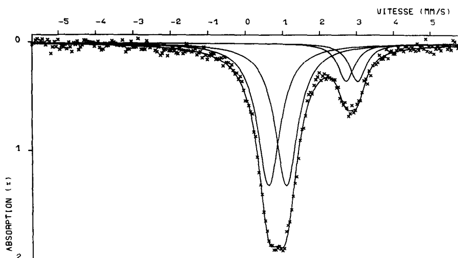
FIG. 3. Spectre Mössbauer à 80 K des polyèdres.
