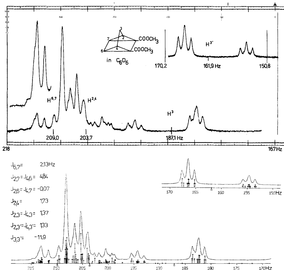
Fig. 3. Experimentelles (oben) und theoretisches 100-MHz-Spektrum (unten) von 18 ( \text{C}_6\text{D}_6 )
