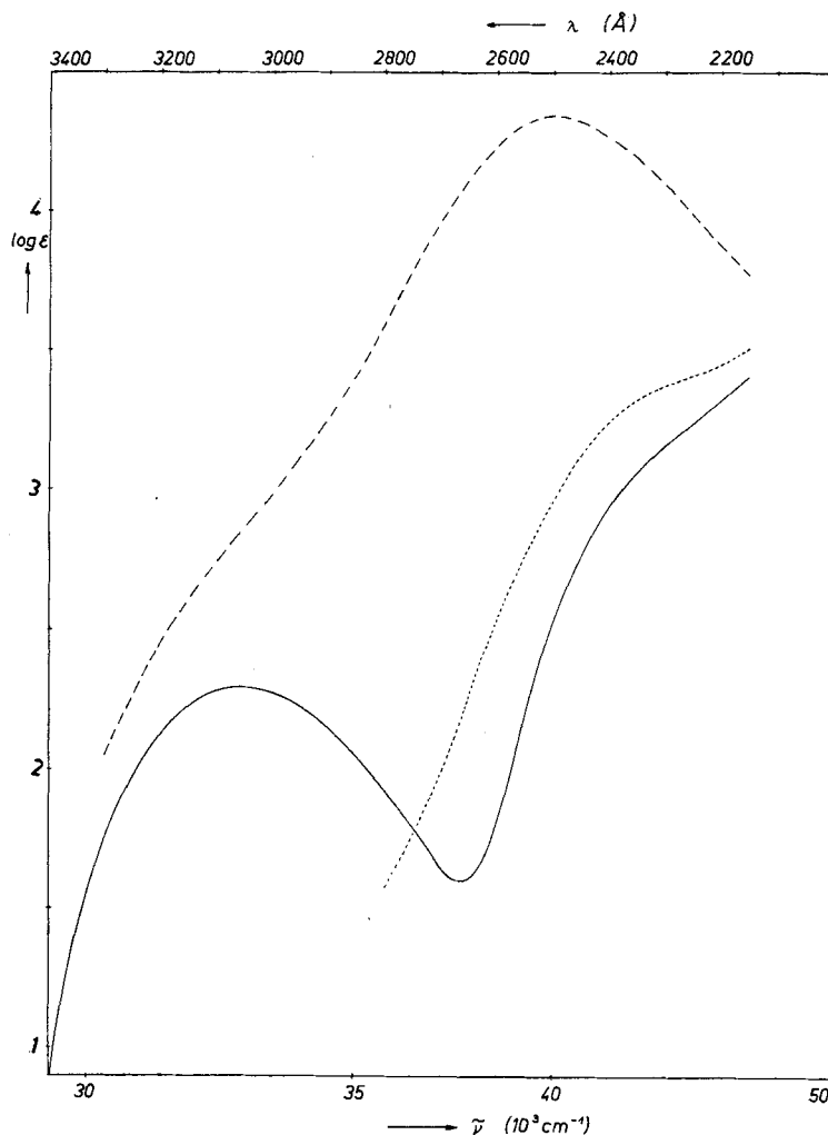
Fig. 2. Elektronenspektren ( \text{CH}_3\text{CN} ) des Ketons 7a (—), des Dicyanmethylenquadricyclans 12a (---) und des Ketals 16a (.....)
