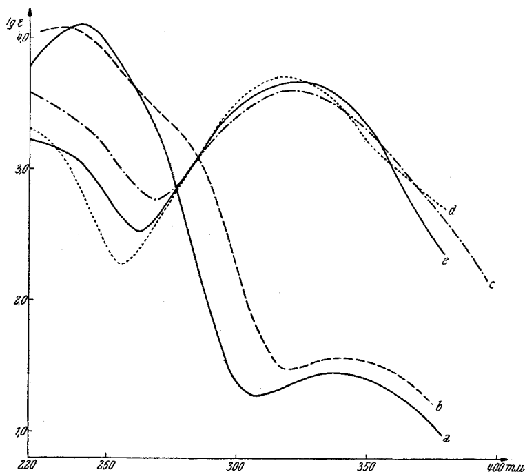
Abb. 3. UV-Absorptionsspektren in Äthanol.
