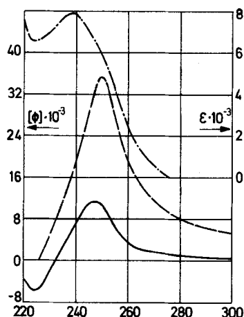
UV.-Absorptionsspektrum (-----) und ORD.-Spektrum (—) von Methyl-(2,3-di-O-benzyl-4-desoxy-4,5-didehydro- \beta -L-threo-hexopyranosid)-uronsäure-methylester (II). – ORD.-Spektrum (—) von Methyl-(2,3-di-O-benzyl-4-desoxy-4,5-didehydro- \alpha -L-threo-hexopyranosid)-uronsäure-methylester.
