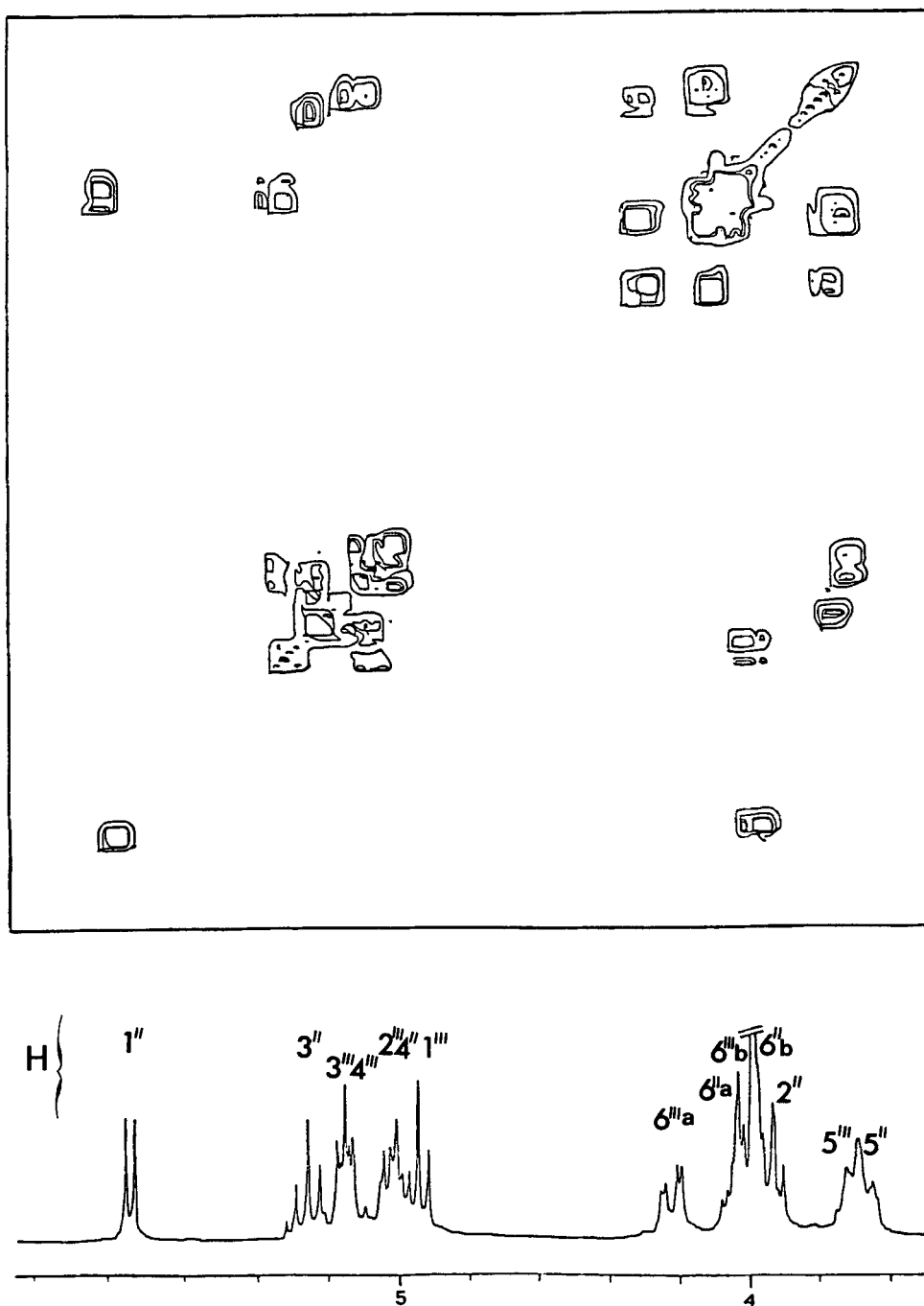
Fig. 2. Spectre de RMN de 2, corrélation ^1\text{H} , ^1\text{H} 2D COSY 90^\circ (270 MHz), région des protons glucidiques (3,60 à 5,80 ppm)
