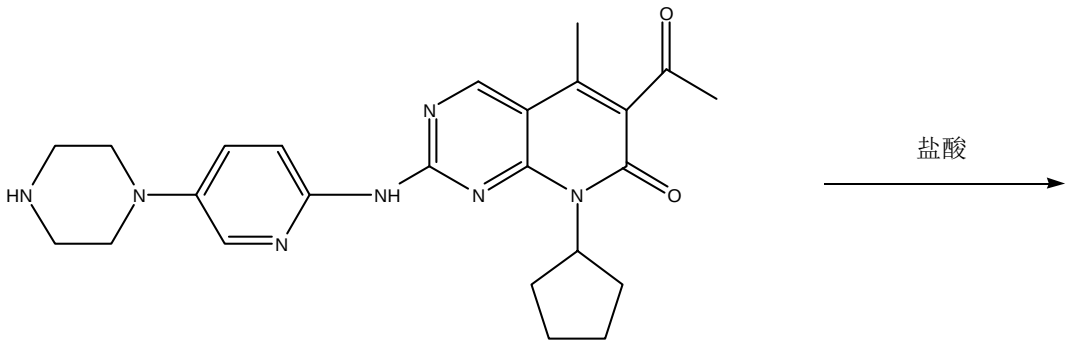
帕布游离碱
