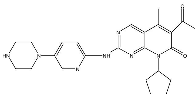
帕布游离碱
