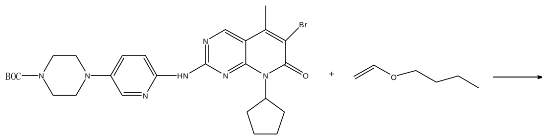
中间体一
