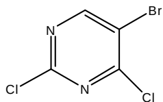
起始原料1
