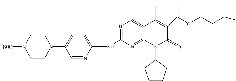
中间体二
