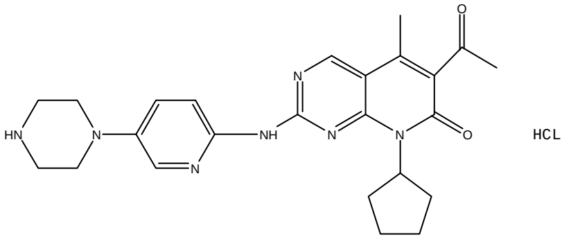
帕布盐酸盐
