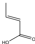
起始原料3
