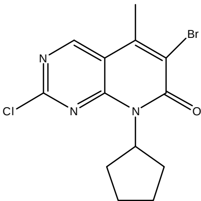
原料二
