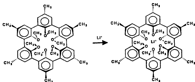
Spheraplex 1\cdot\text{Li}^+
